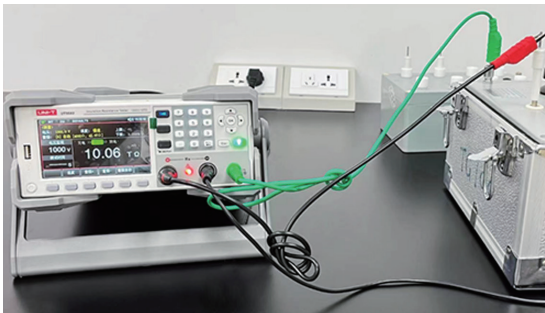
电阻测试范围10kΩ~10TΩ
