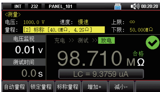
标称量程设置,根据比较器设定自动选择量程
